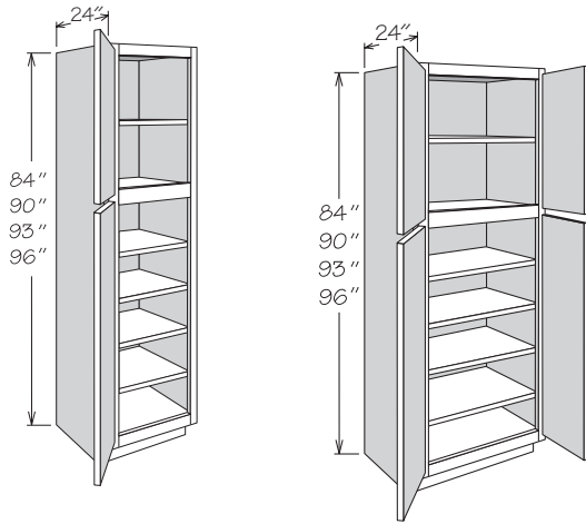
2 DOORS
