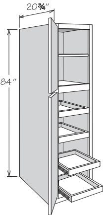
2 DOOR
